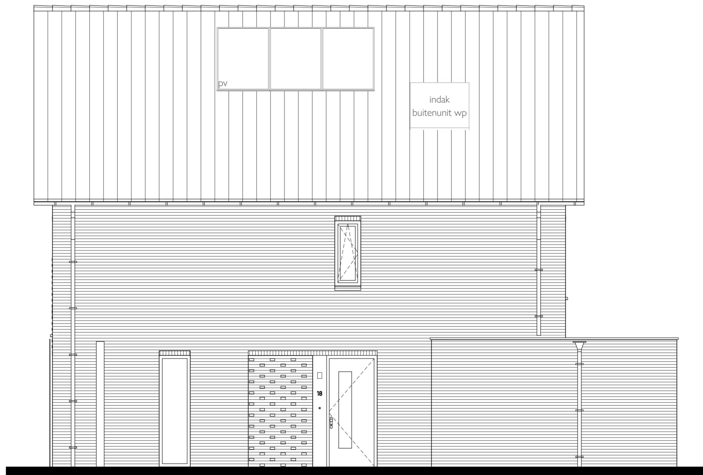
Rechtergevel
