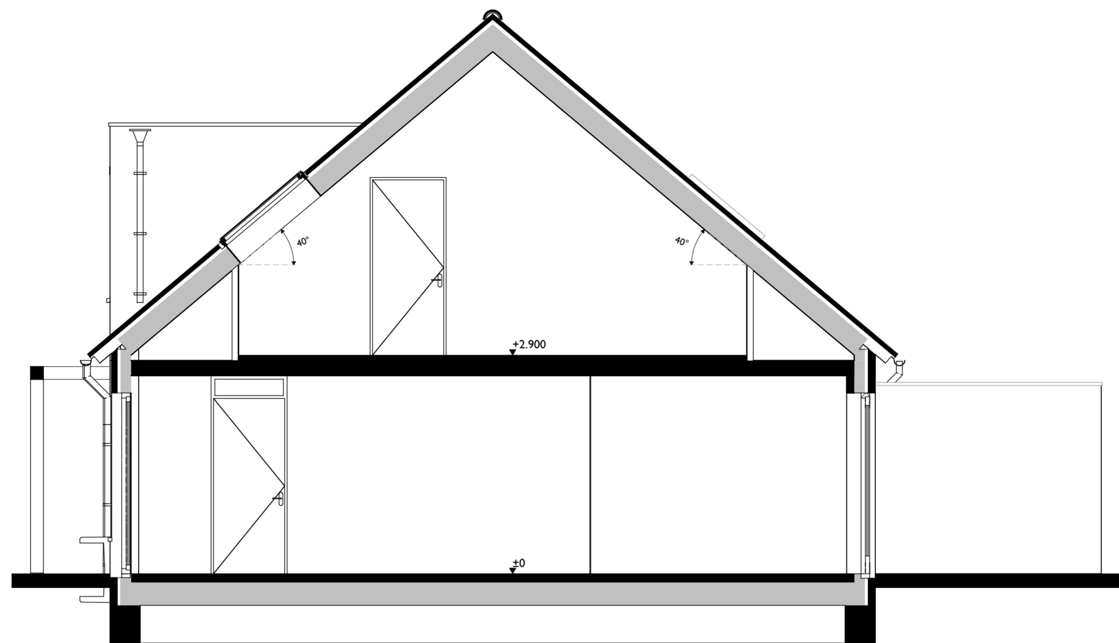
Doorsnede
