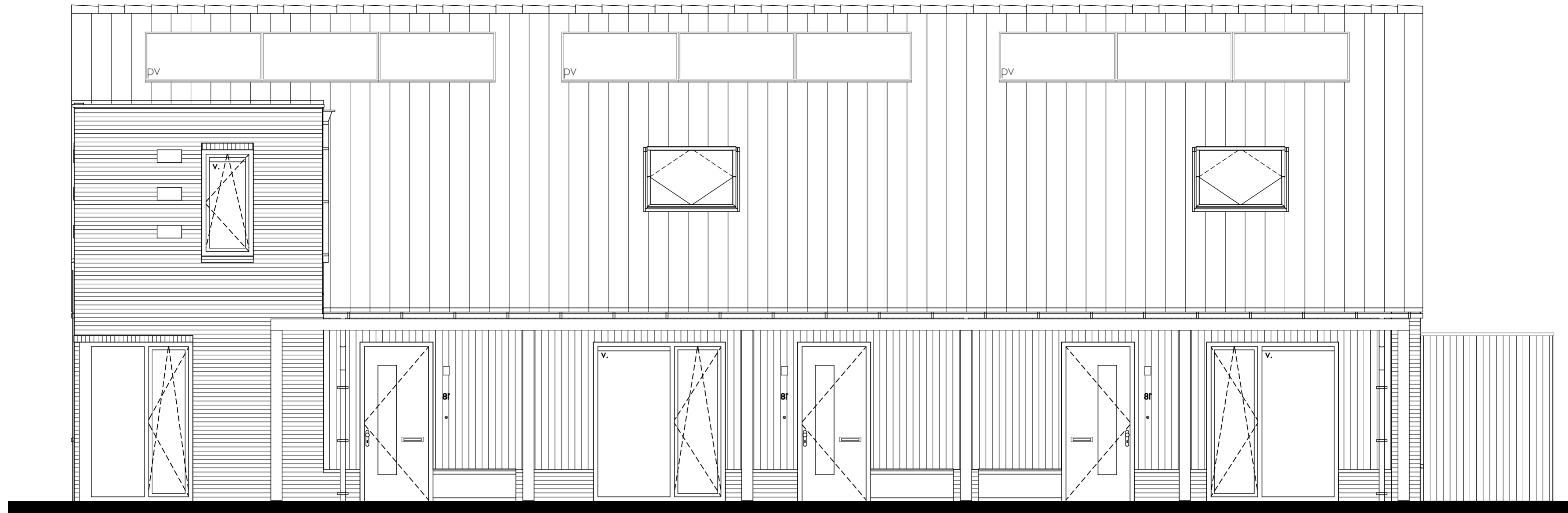
Voorgevel (zuid)
