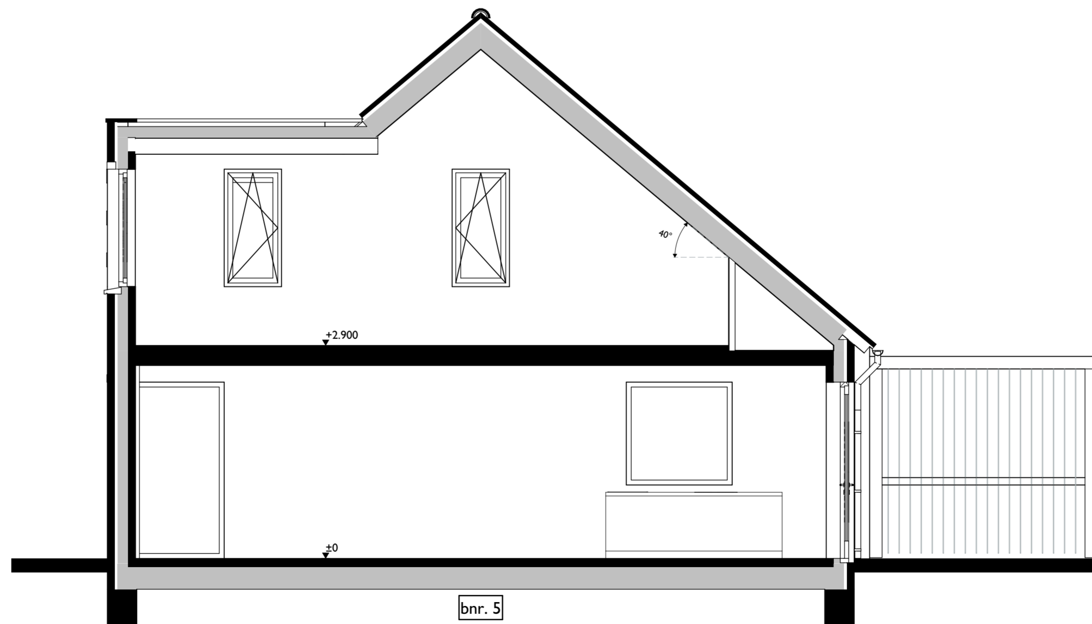
Doorsnede kopwoning
