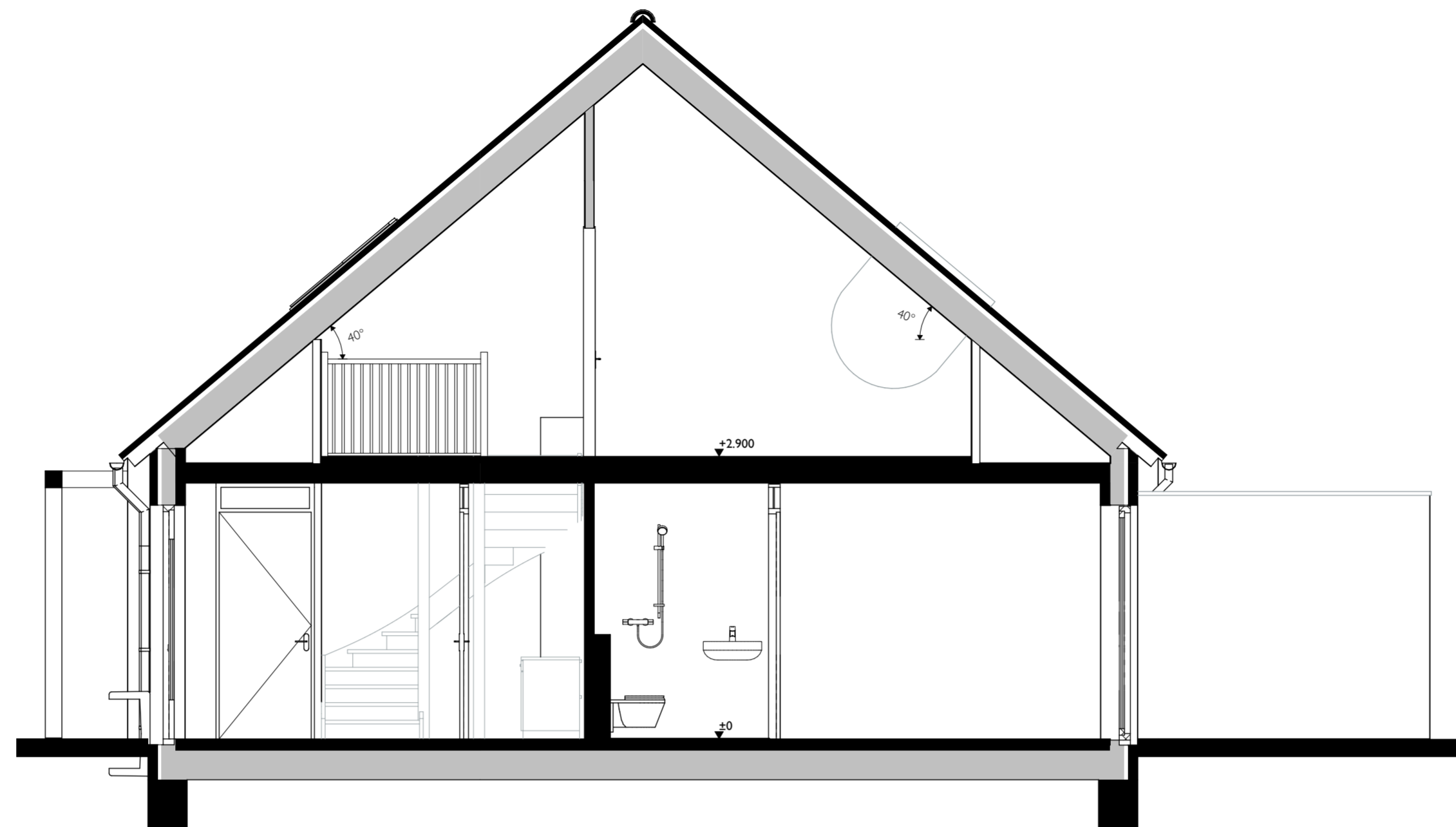
Doorsnede
