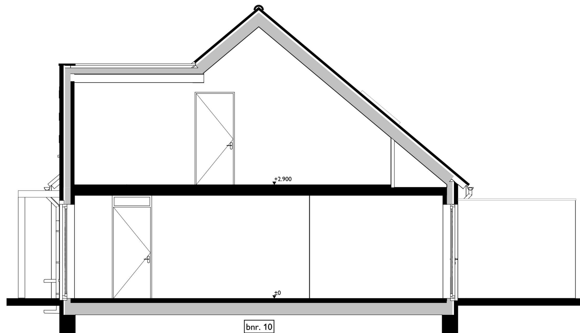
Doorsnede kopwoning
