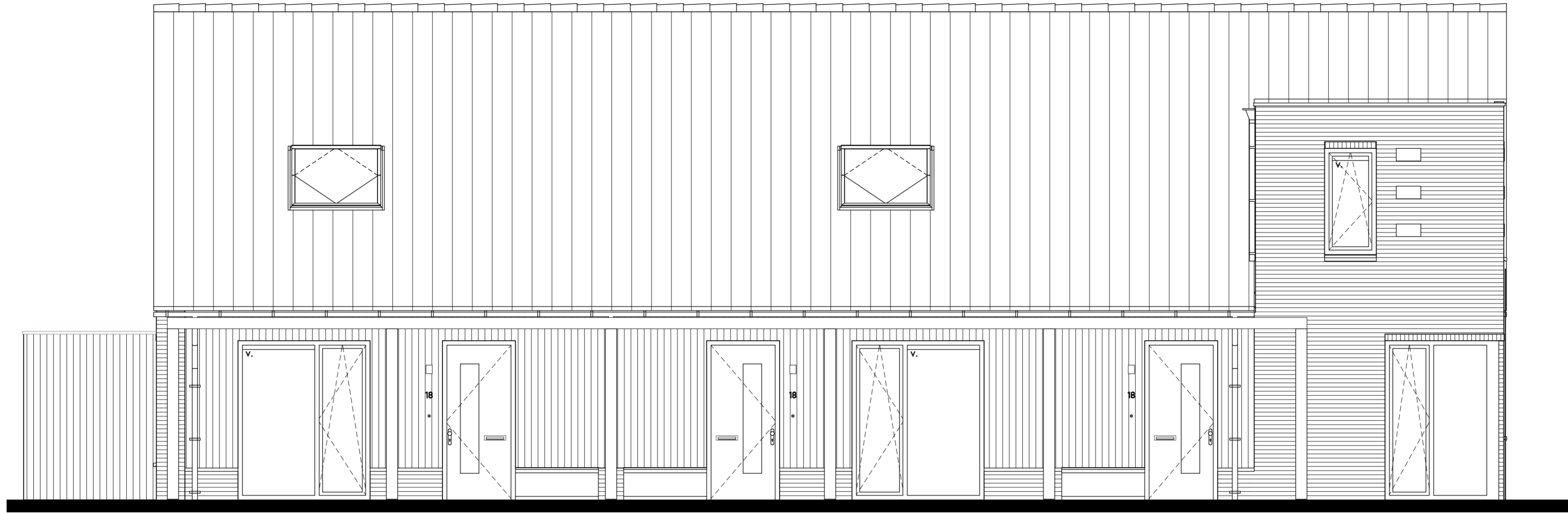
Voorgevel (noord)
