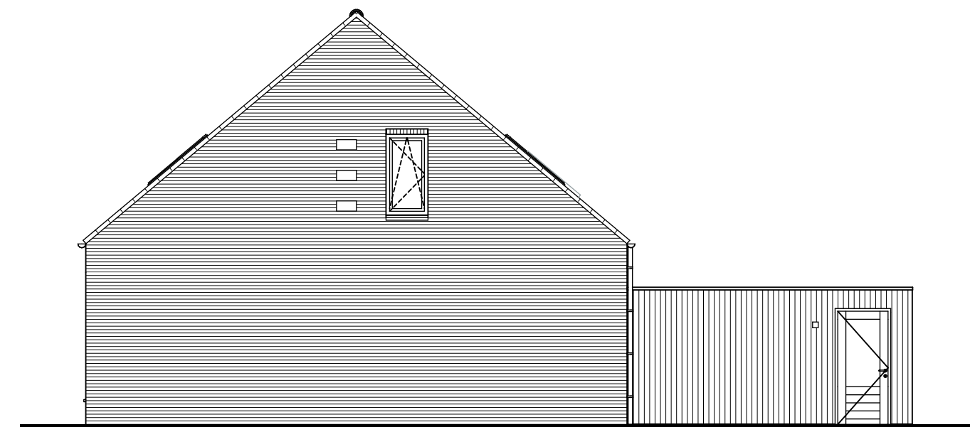
Rechtergevel
