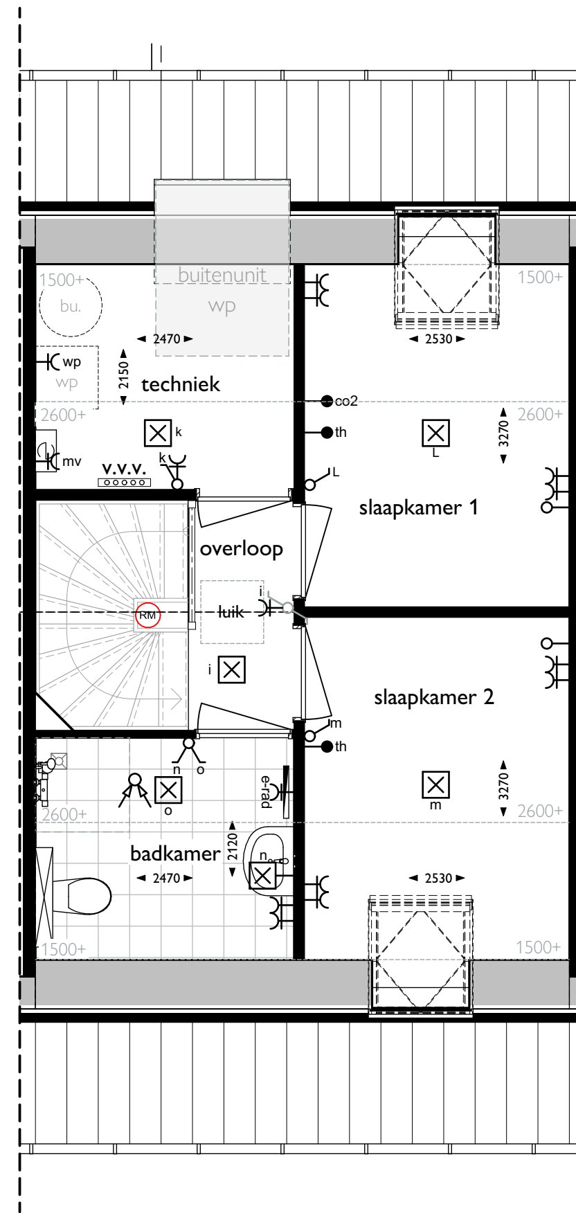
01 eerste verdieping
