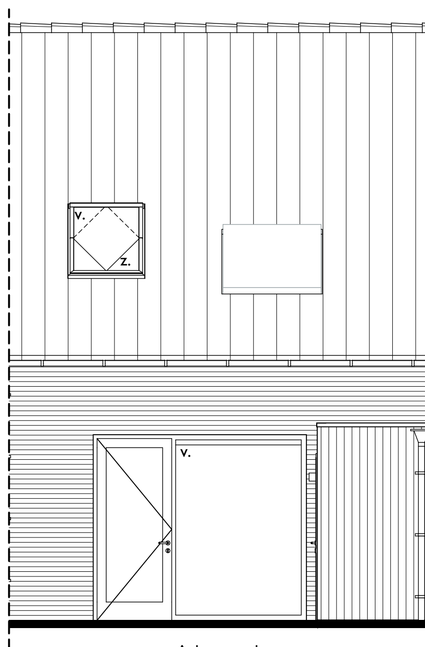
Achtergevel
