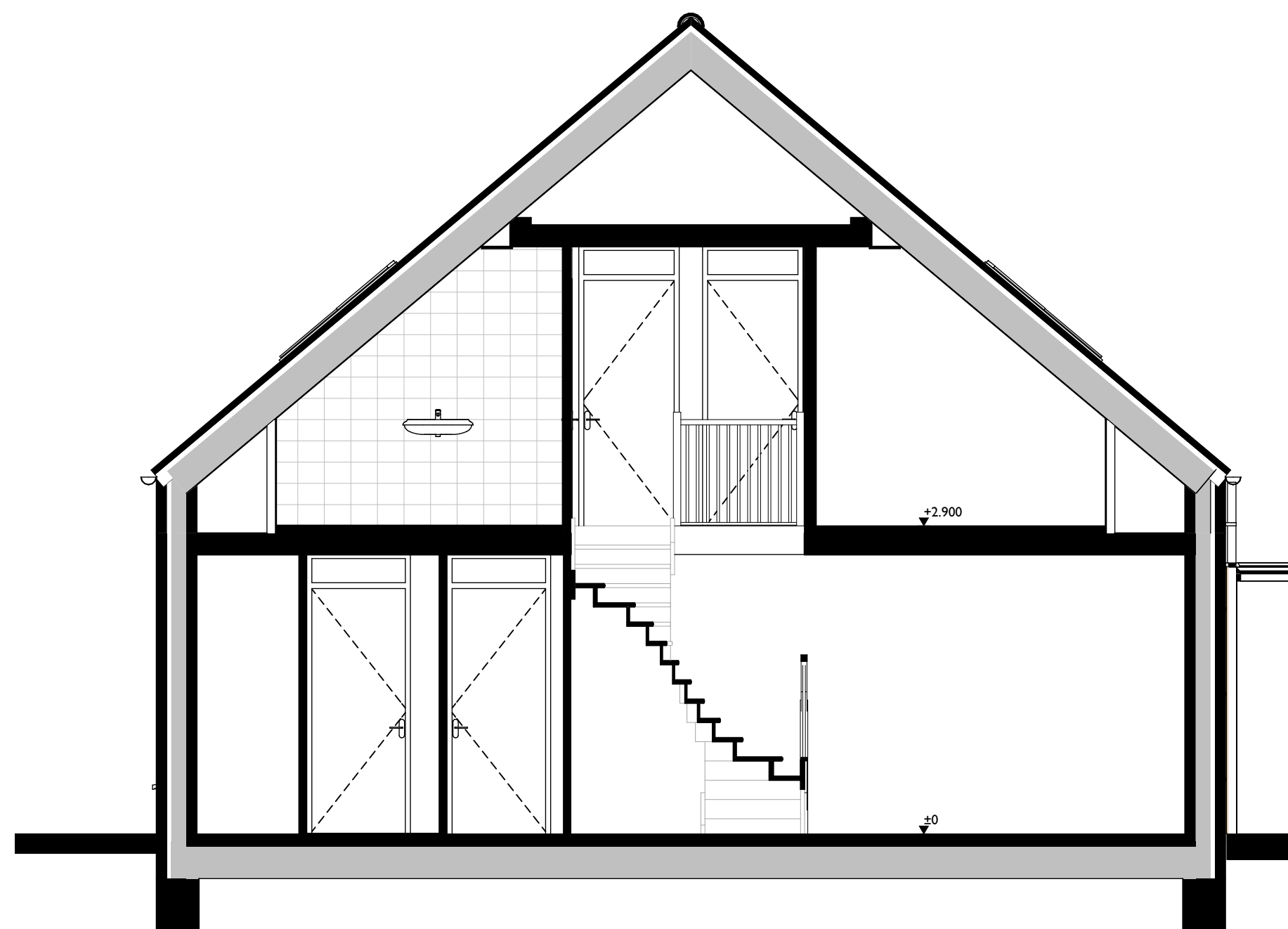
Doorsnede
