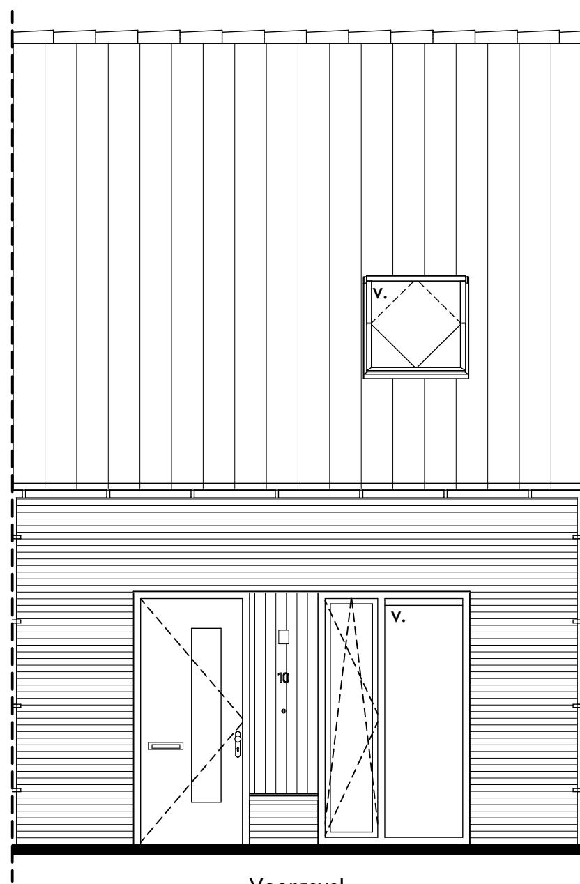
Voorgevel
