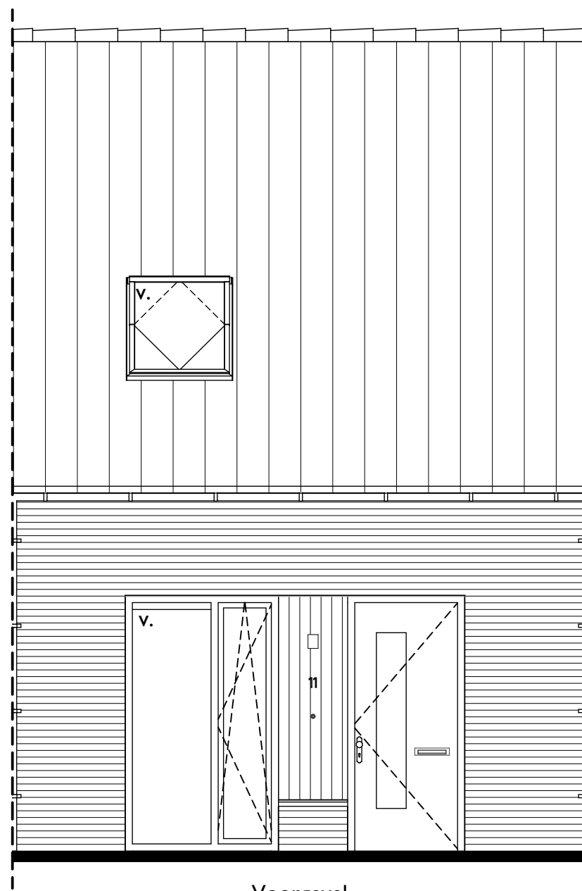
Voorgevel
