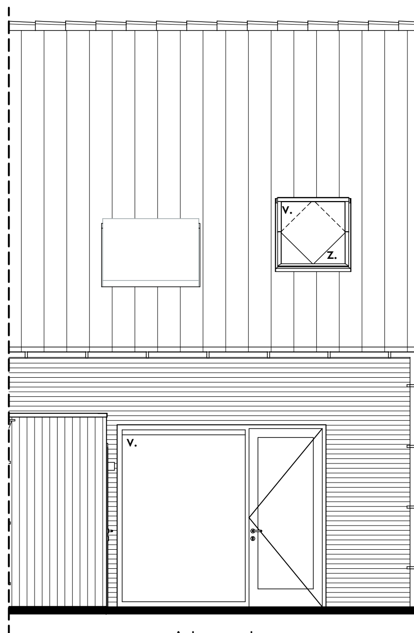
Achtergevel
