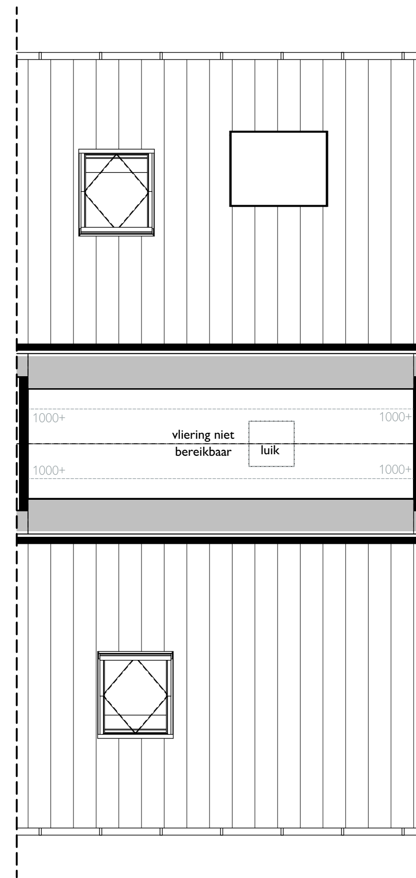
02 vleringzolder
