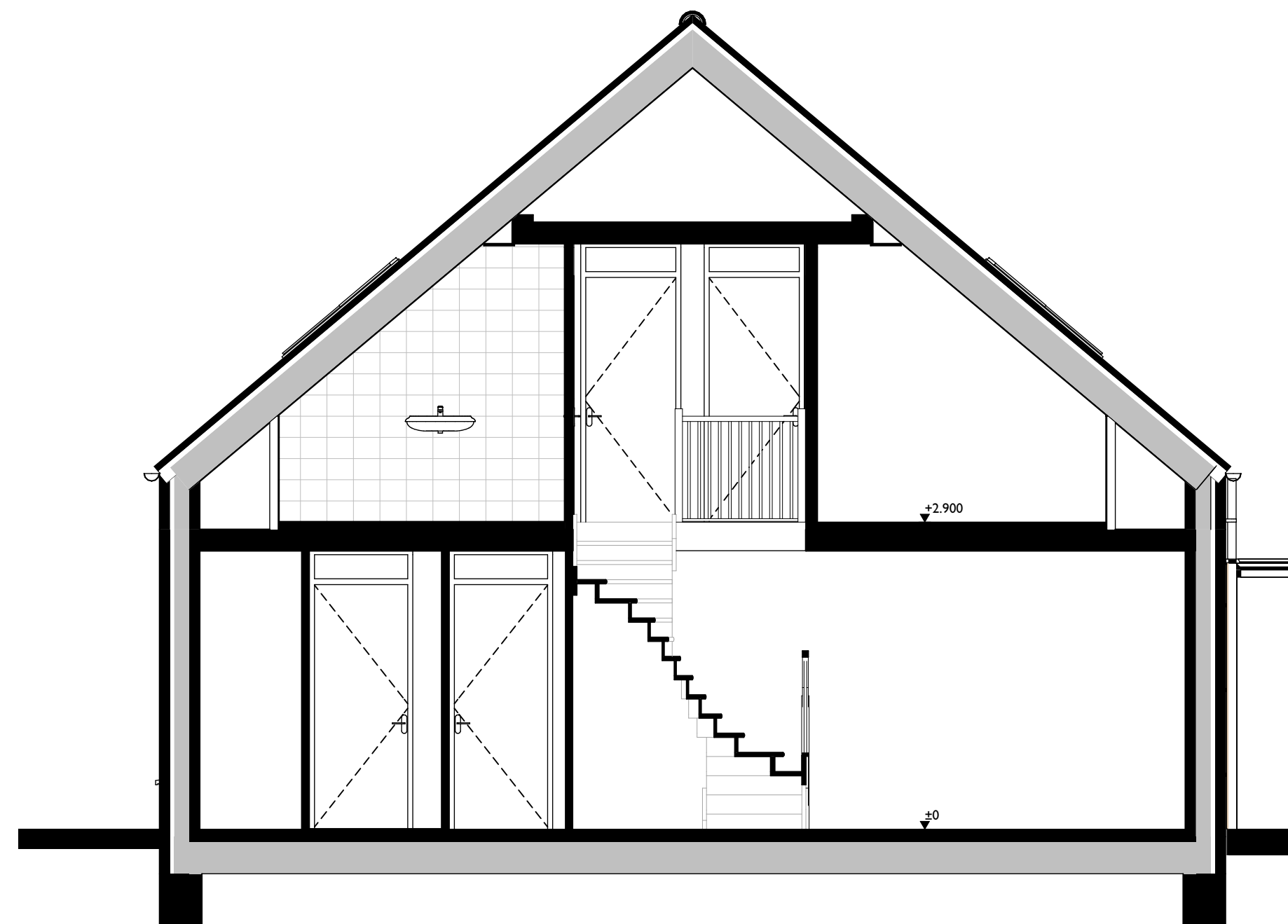
Doorsnede
