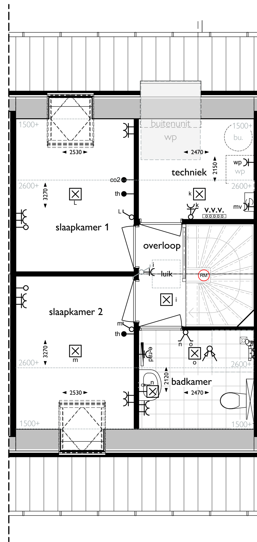
01 eerste verdieping
