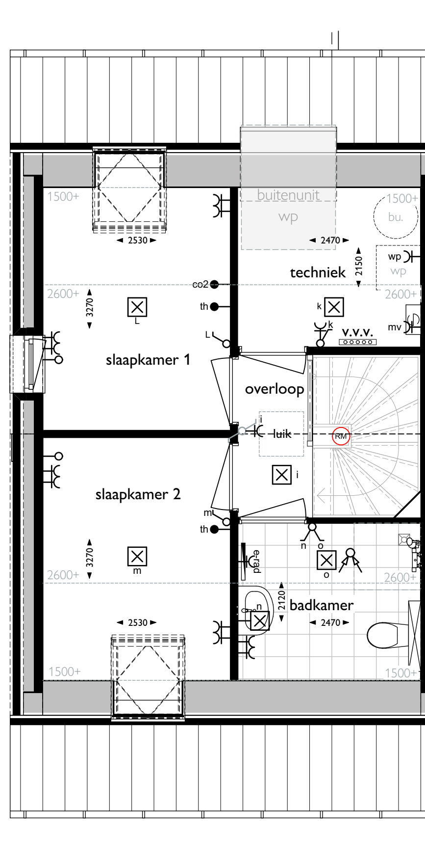
01 eerste verdieping
