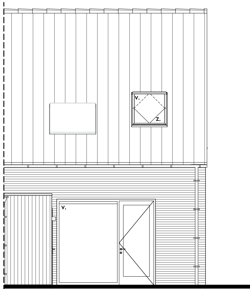
Achtergevel
