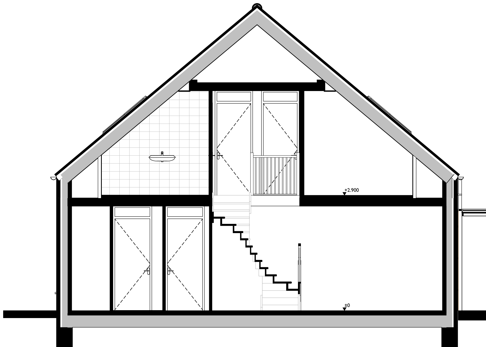
Doorsnede
