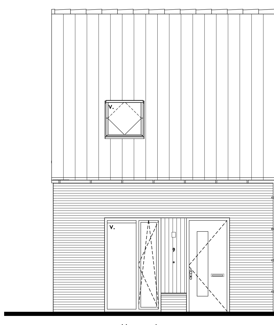
Voorgevel
