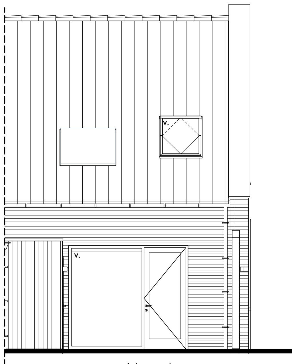
Achtergevel
