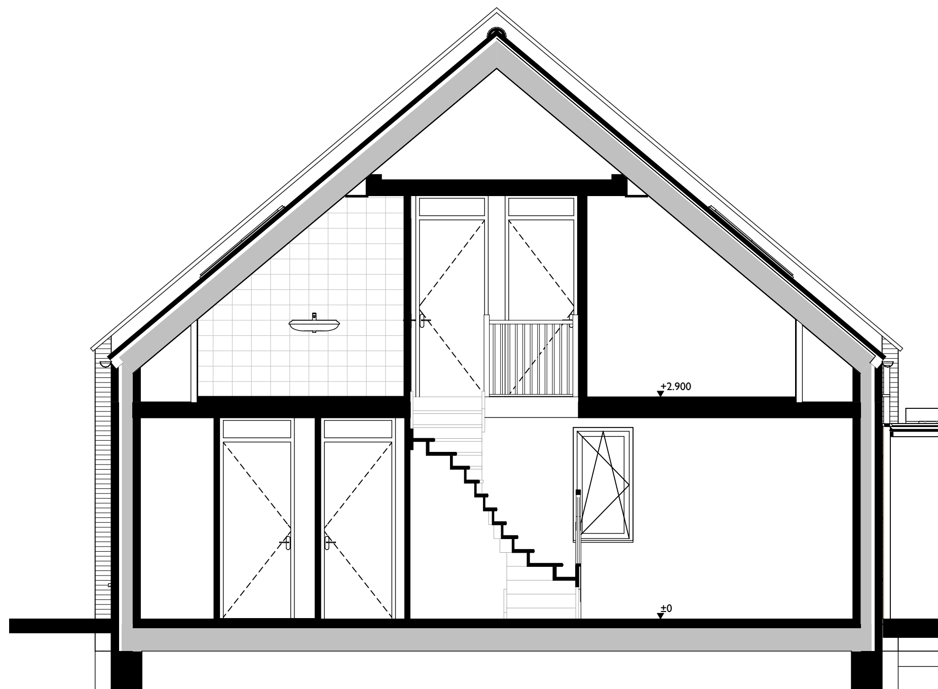
Doorsnede
