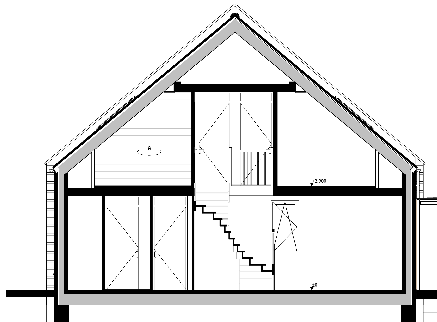
Doorsnede
