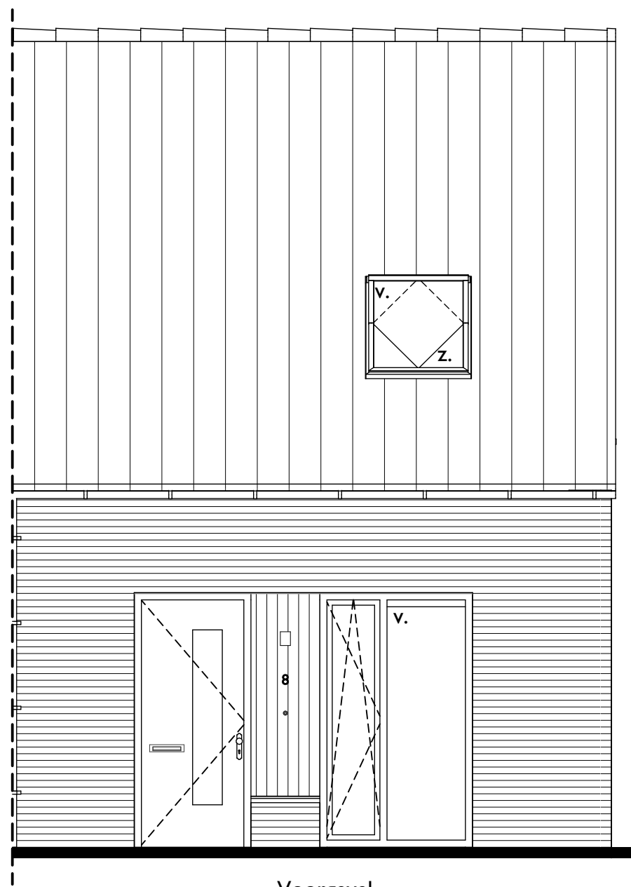
Voorgevel
