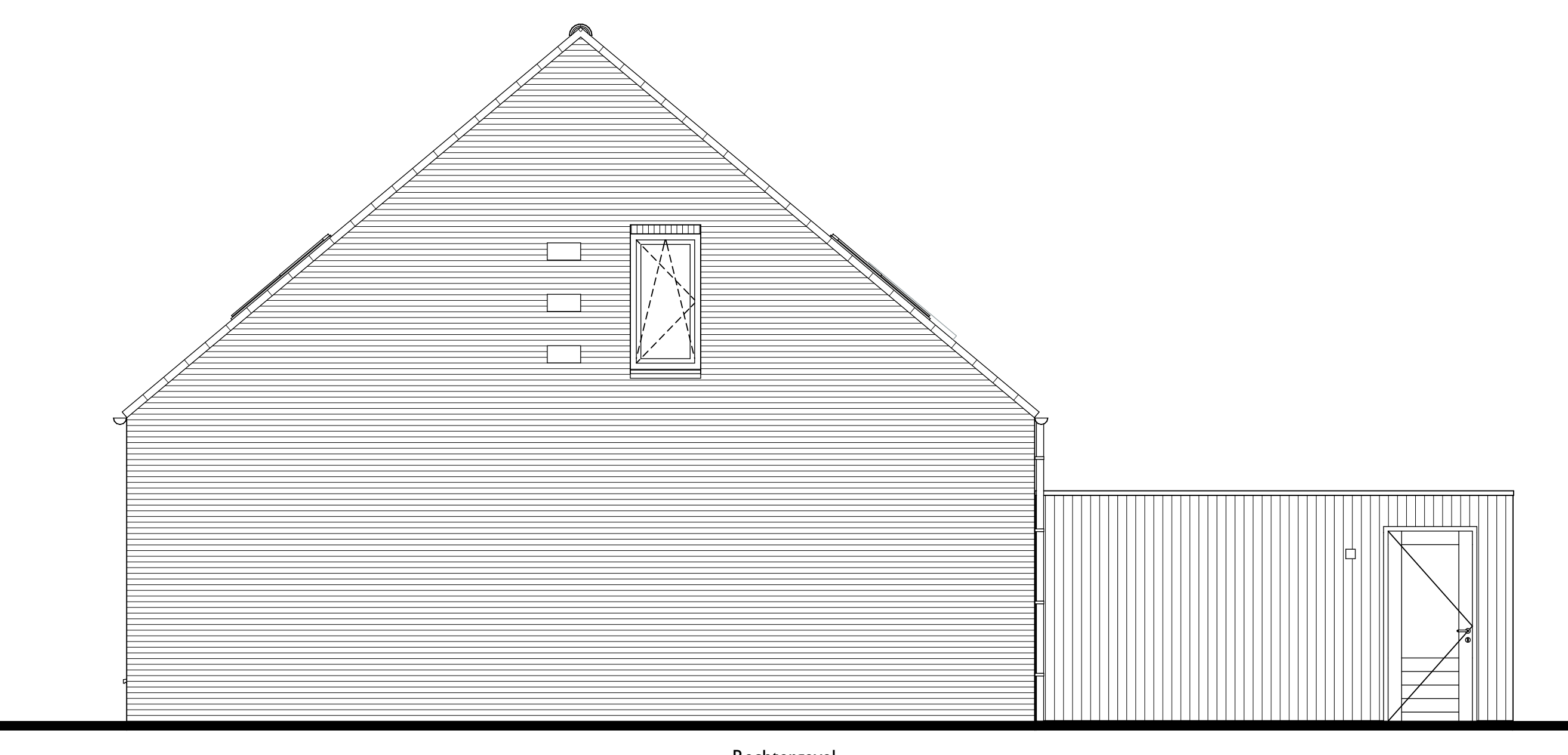
Rechtergevel
