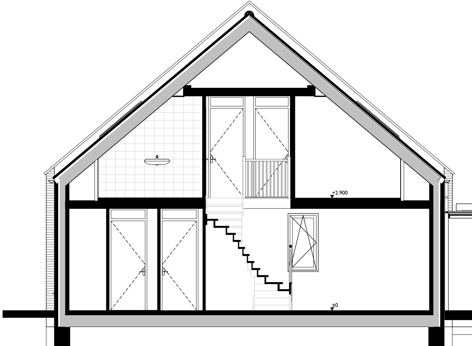
Doorsnede
